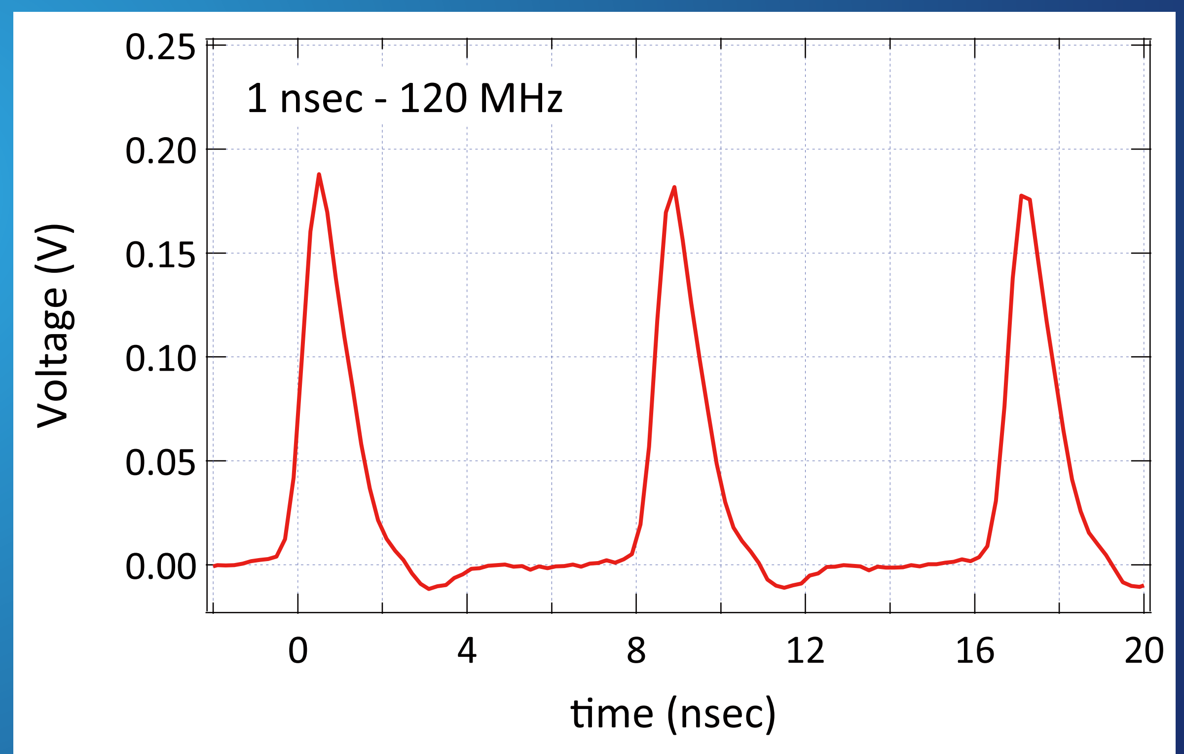
パルス出力の時間プロフィール
