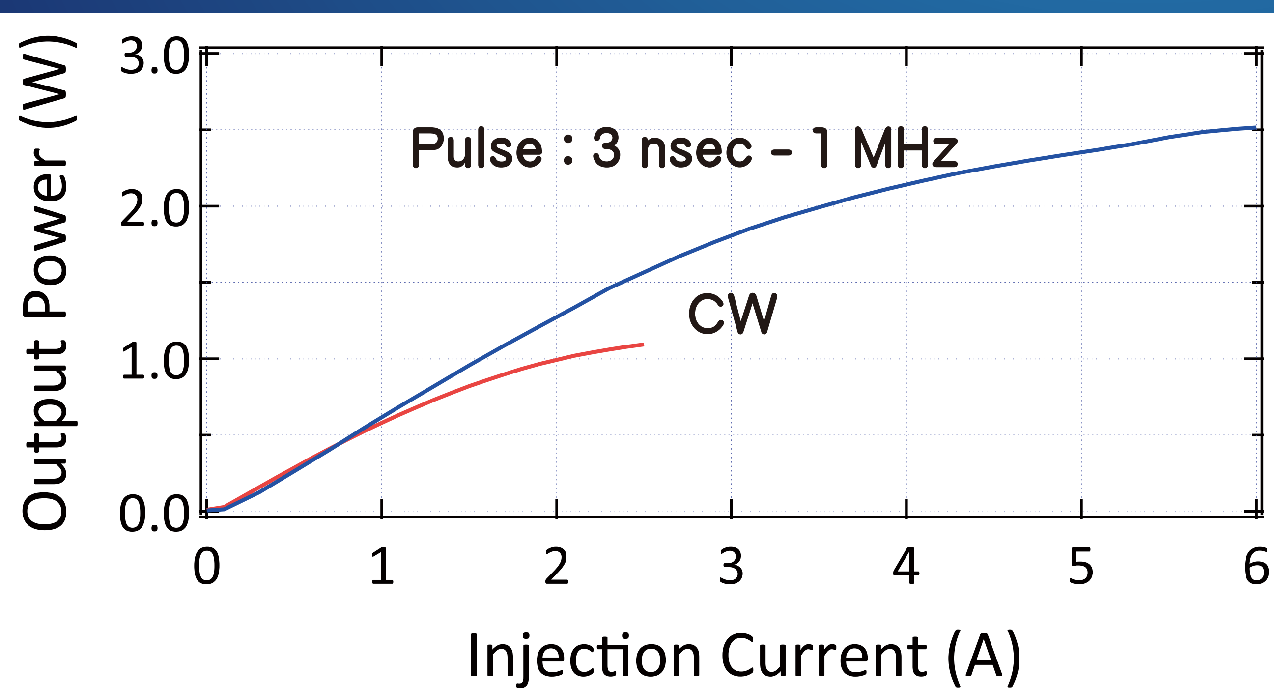
パルス出力の注入電流特性
