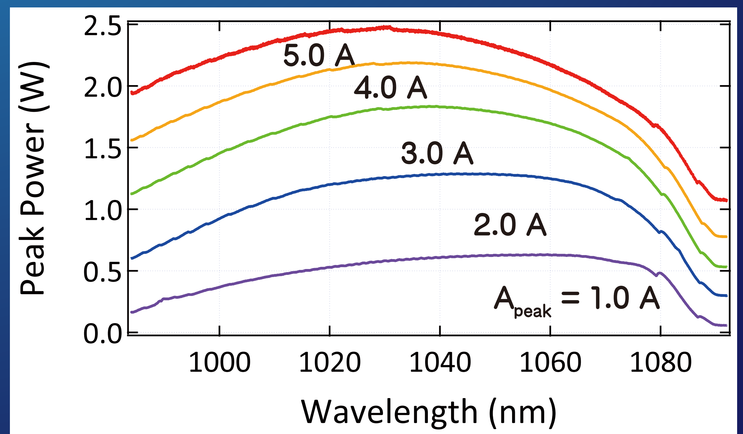
パルス出力の入力波長特性
