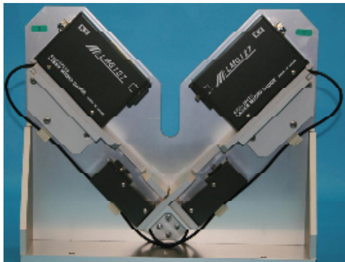
分離式XY測定用架台
