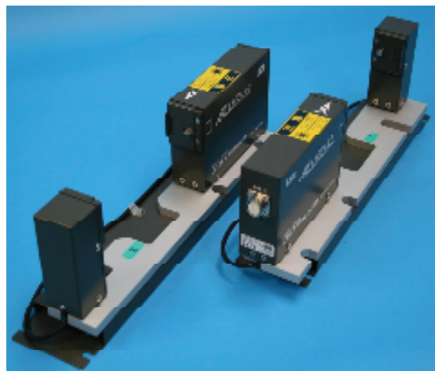
分離式XY測定用架台
