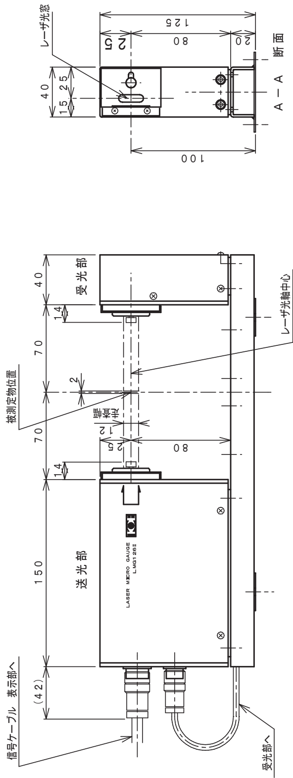
LMG126II センサ部
