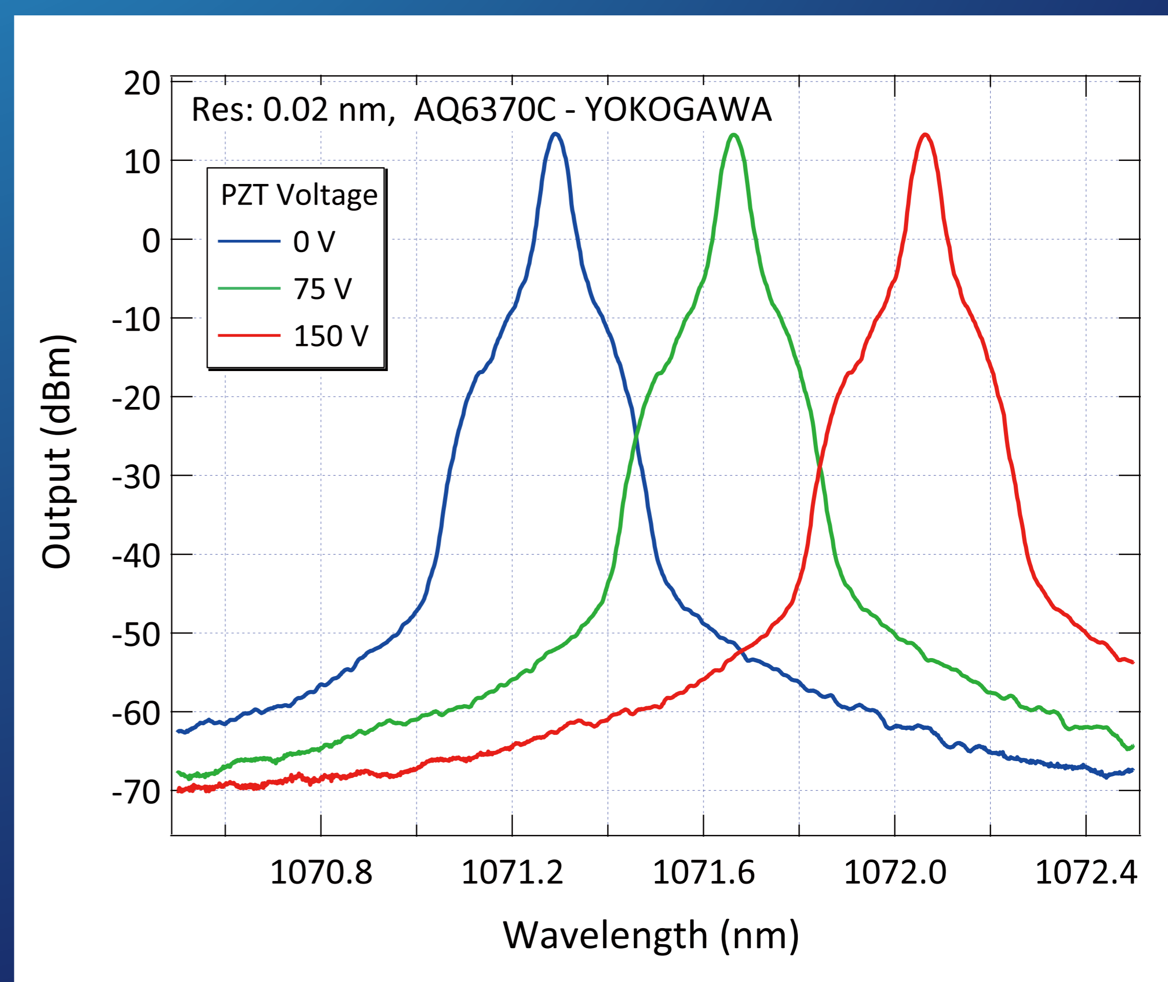
狭線幅・ASE-Free 発振特性
