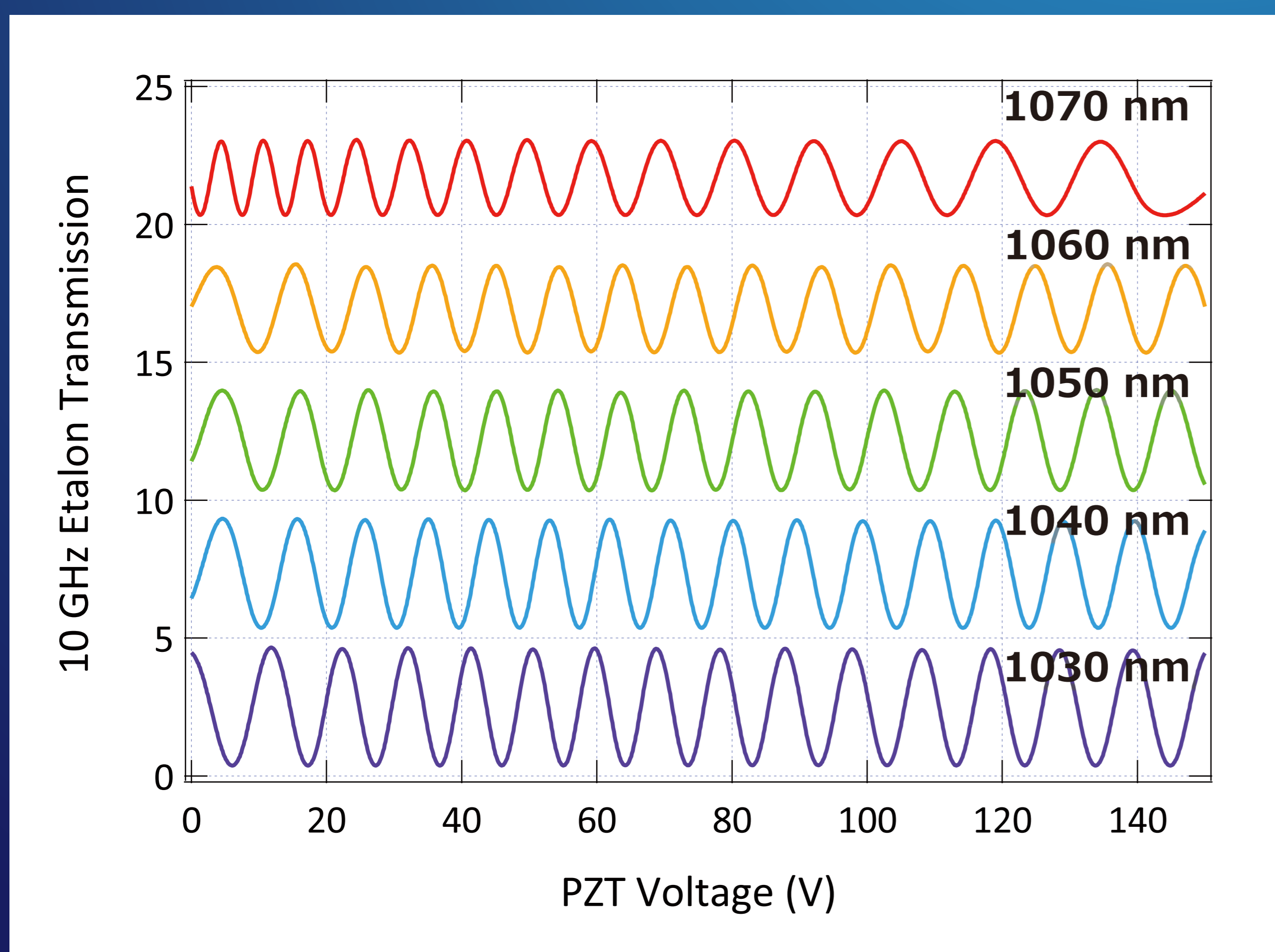
各波長でのモードホップフリー掃引特性
